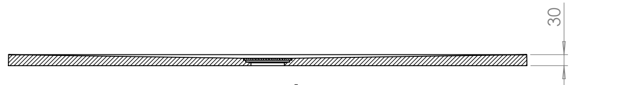
PRZEKRÓJ A-A
